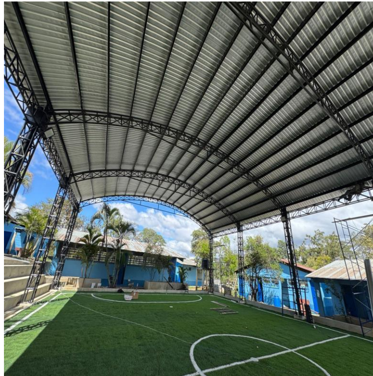
MEJORAMIENTO ESCUELA PRIMARIA ALDEA SAN RAFAEL RABINAL, BAJA VERAPAZ. SNIP 315707 AVANCE FÍSICO 100%
